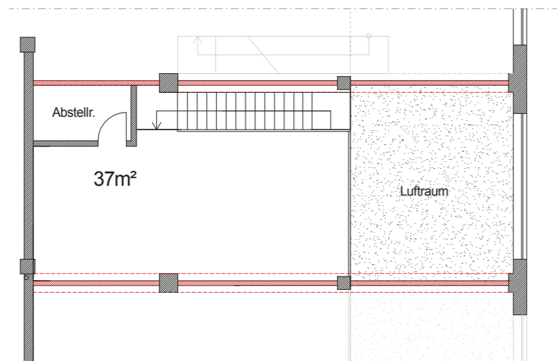
Galerie
