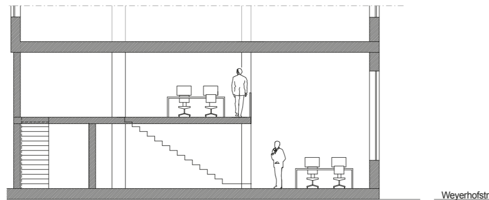
Schemaschnitt
