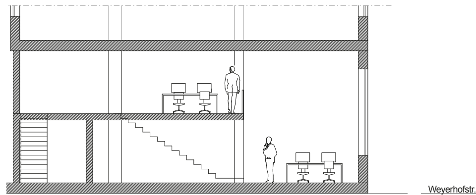
Schemaschnitt
