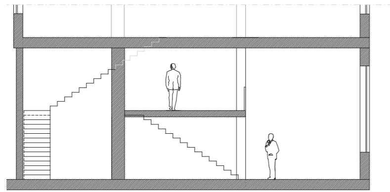
Schemaschnitt
