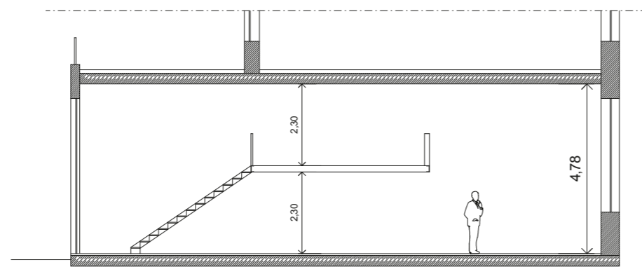
Schemaschnitt
