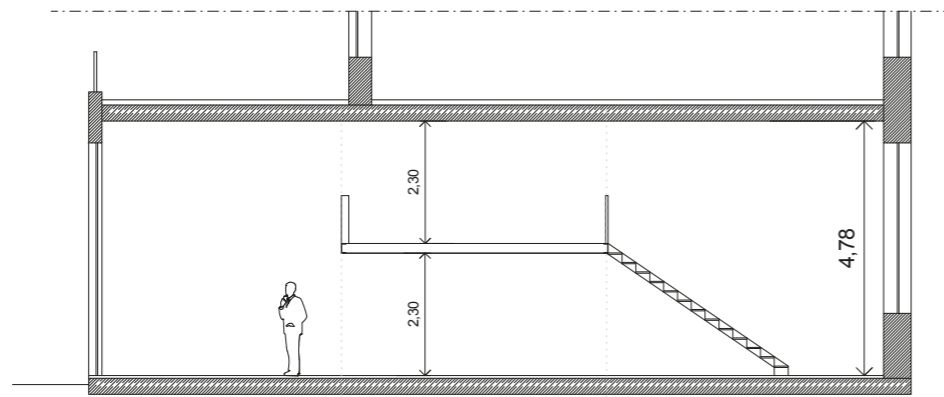
Schemaschnitt
