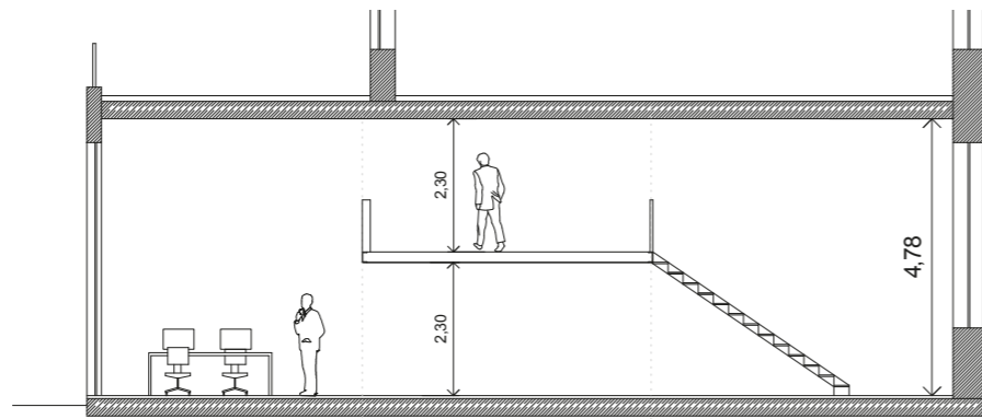
Schemaschnitt
