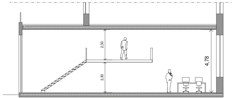
Schemaschnitt
