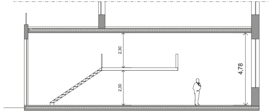
Schemaschnitt
