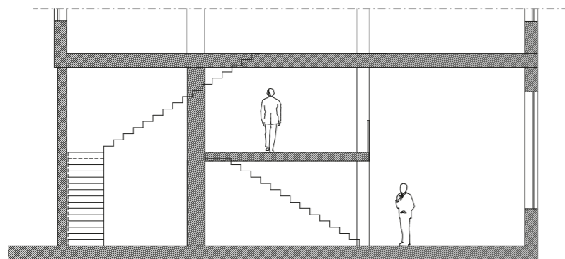
Schemaschnitt
